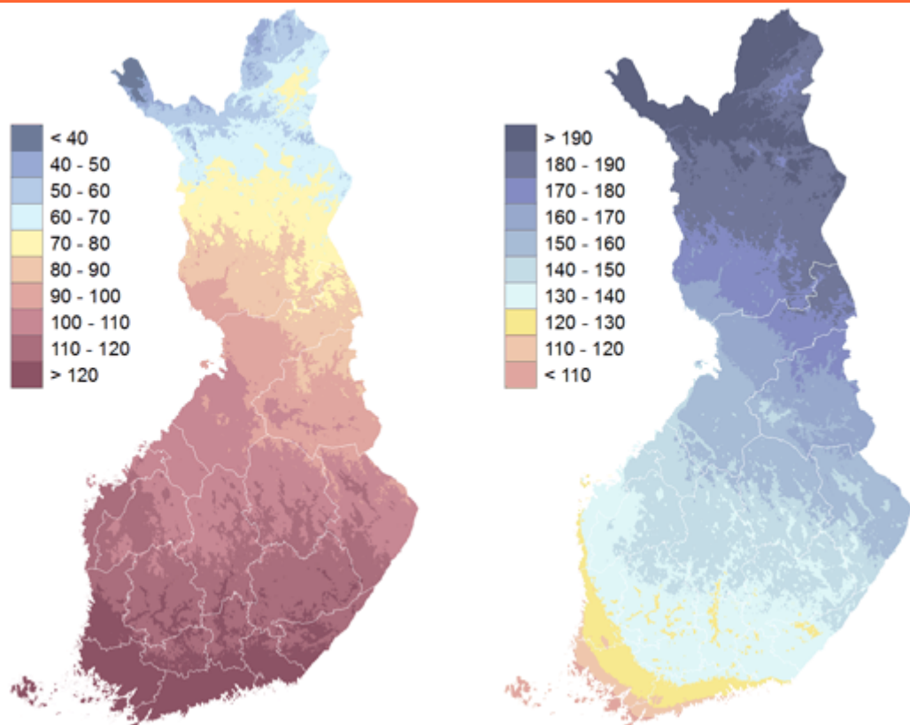
Kuva 6-4 Keskimääräinen kesän pituus vuorokausina (vasemmalla) sekä talven pituus (oikealla) vertailukaudella 1981–2010 (Ilmatieteen laitos 2016b).
